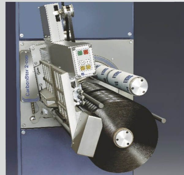
Automatischer Take-up 2-cop Spuler für Karbonfasern und Towpreg
